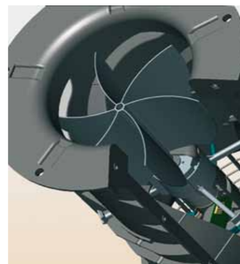
1 Вентилятор VBP в разрезе
