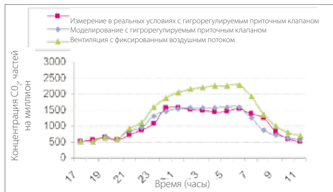
Рисунок 2: Изменение концентрации CO 2 ночью 3 . Сравнение гиррорегулируемого приточного воздушного клапана (измеренного и смоделированного) и вентиляции с фиксированным потоком (смоделированной).
