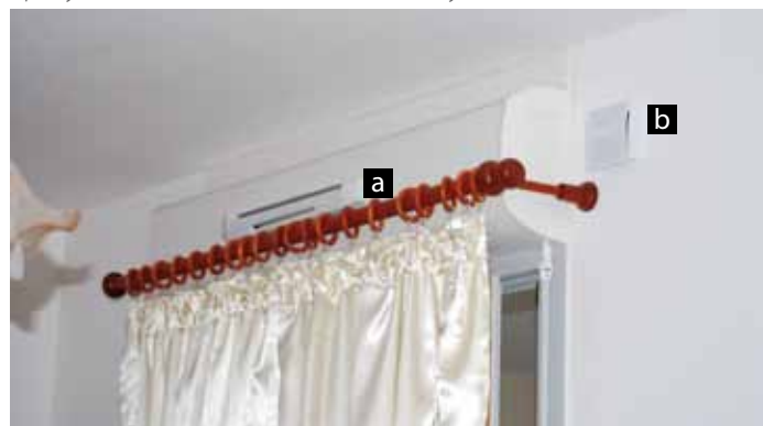
Гигрорегулируемое приточное устройство Аэрэко на рольставнях (a). Датчик влажности, температуры воздуха и концентрации CO_2 (b).
