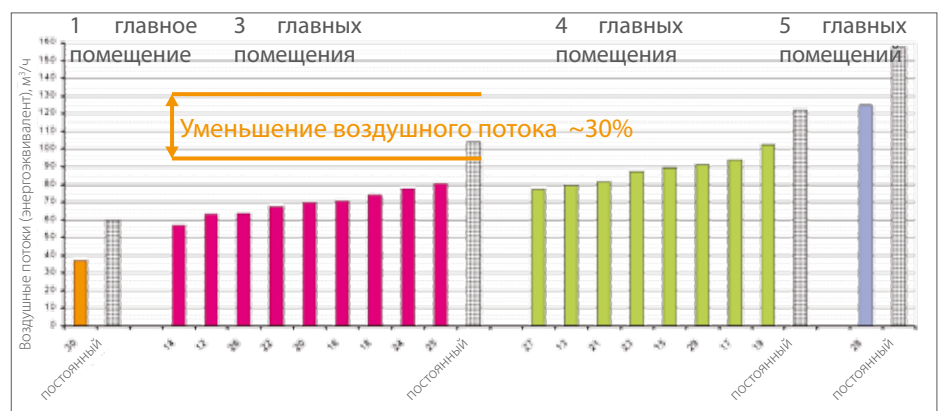
Рисунок 4: Статистический энергоэквивалент воздушного потока в расчете на квартиру в г. Париже. Поделен по типам квартир в соответствии с французскими нормативами постоянного воздушного потока. Отопительный период 2008-2009.
